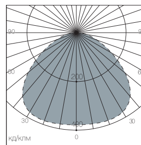
DOLO 70/G12
