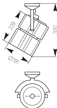
DOLO 70
